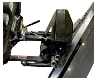
Elhydraulisk enhet
